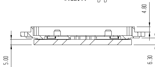
Schnitt B-B
